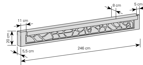
Płyta 20 podmurówka z okapnikiem
