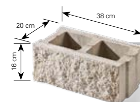
Pustak łupany „wpust-wypust”
