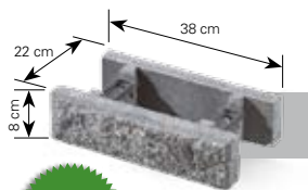
Pustak z kształtek (podmurówkowy)
