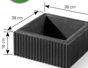
Pustak ryflowany (słupkowy)
