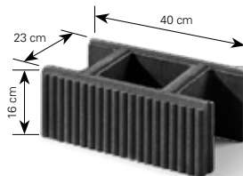
Pustak ryflowany (podmurówkowy)
