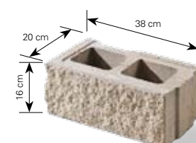
Pustak łupany narożny (prawy)
