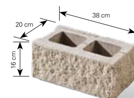
Pustak łupany narożny (lewy)
