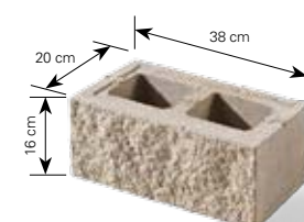
Pustak łupany końcowy „bez wpustu”
