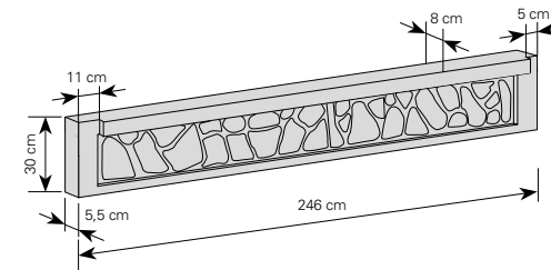
Płyta 30 podmurówka z okapnikiem
